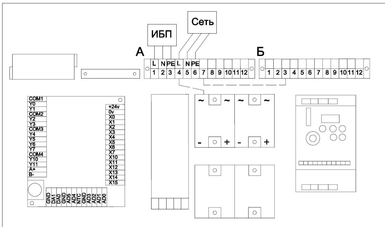
Рис. 8 Блок управления
