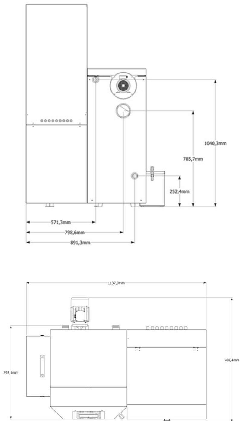
Рис. 5 - Габаритные размеры котла
