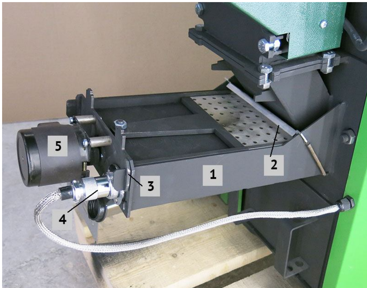
1. Горелка. 2. Скрепер. 3. Фиксатор. 4. Разъем. 5. Электродвигатель 6.
