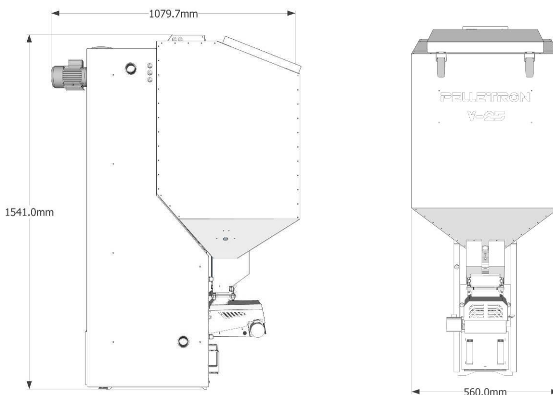
Габаритные размеры котла Pelletron-V25i с бункером 250 л.
