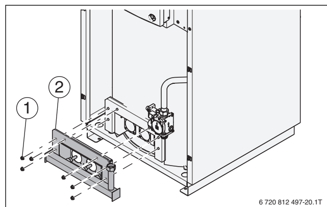
Рис. 33 Отверните крепёжные гайки
