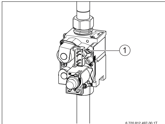
Рис. 21 Удаление воздуха из газопровода
