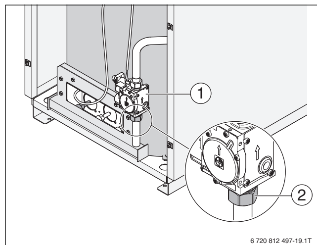
Рис. 32 Демонтаж горелки
