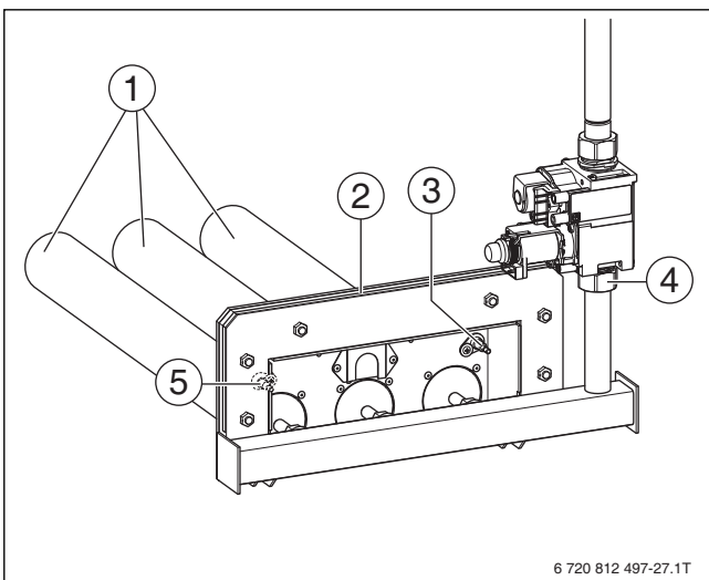
Рис. 37 Чистка горелки
