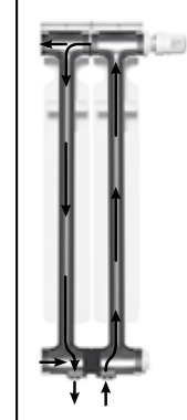
Рисунок 1.3. Вид радиатора RADENA BIMETALL VC500
