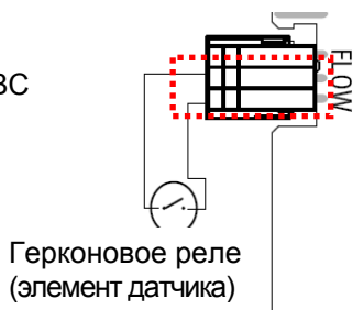
Герконовое реле
