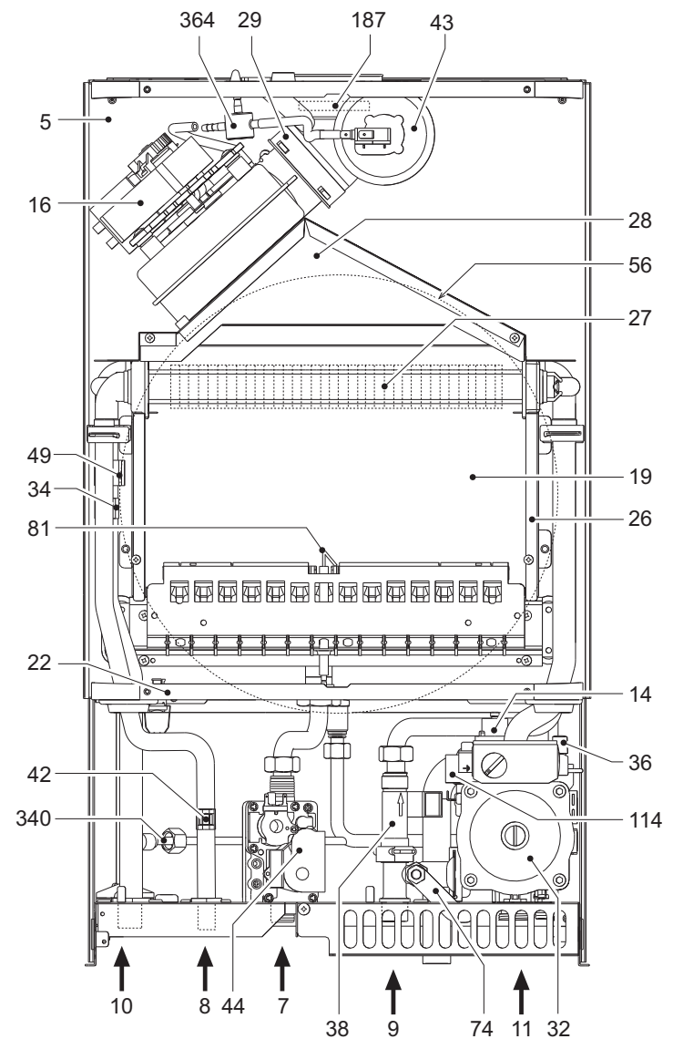
рис. 17 - Общий вид
