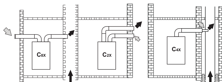
рис. 11 - Примеры подсоединения к дымоходам (⇨ = Воздух / ⇨ = Дымовые газы)
