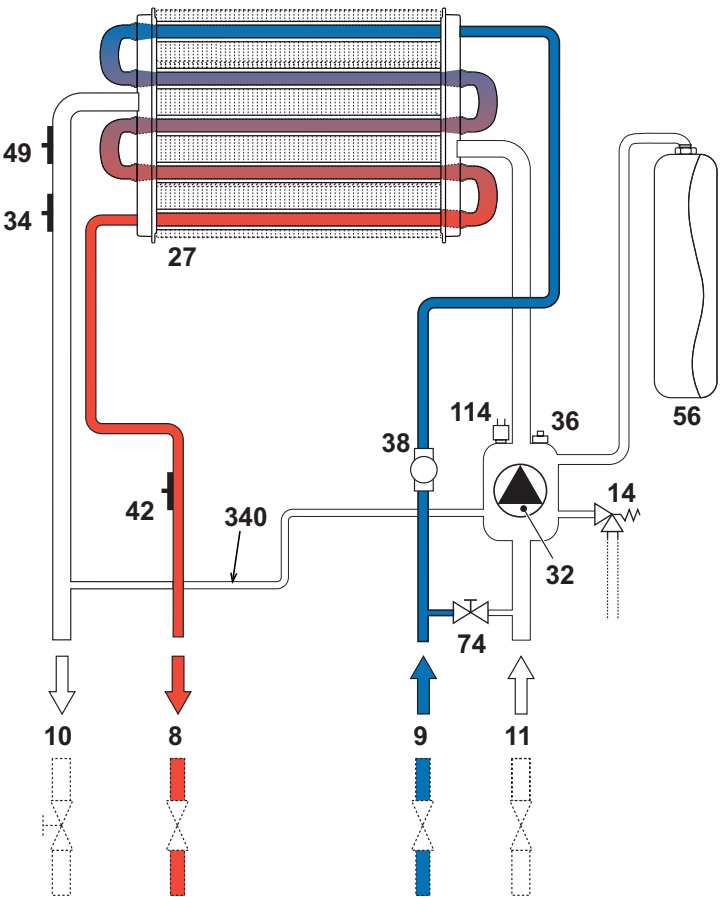
рис. 19 - Контур ГВС
