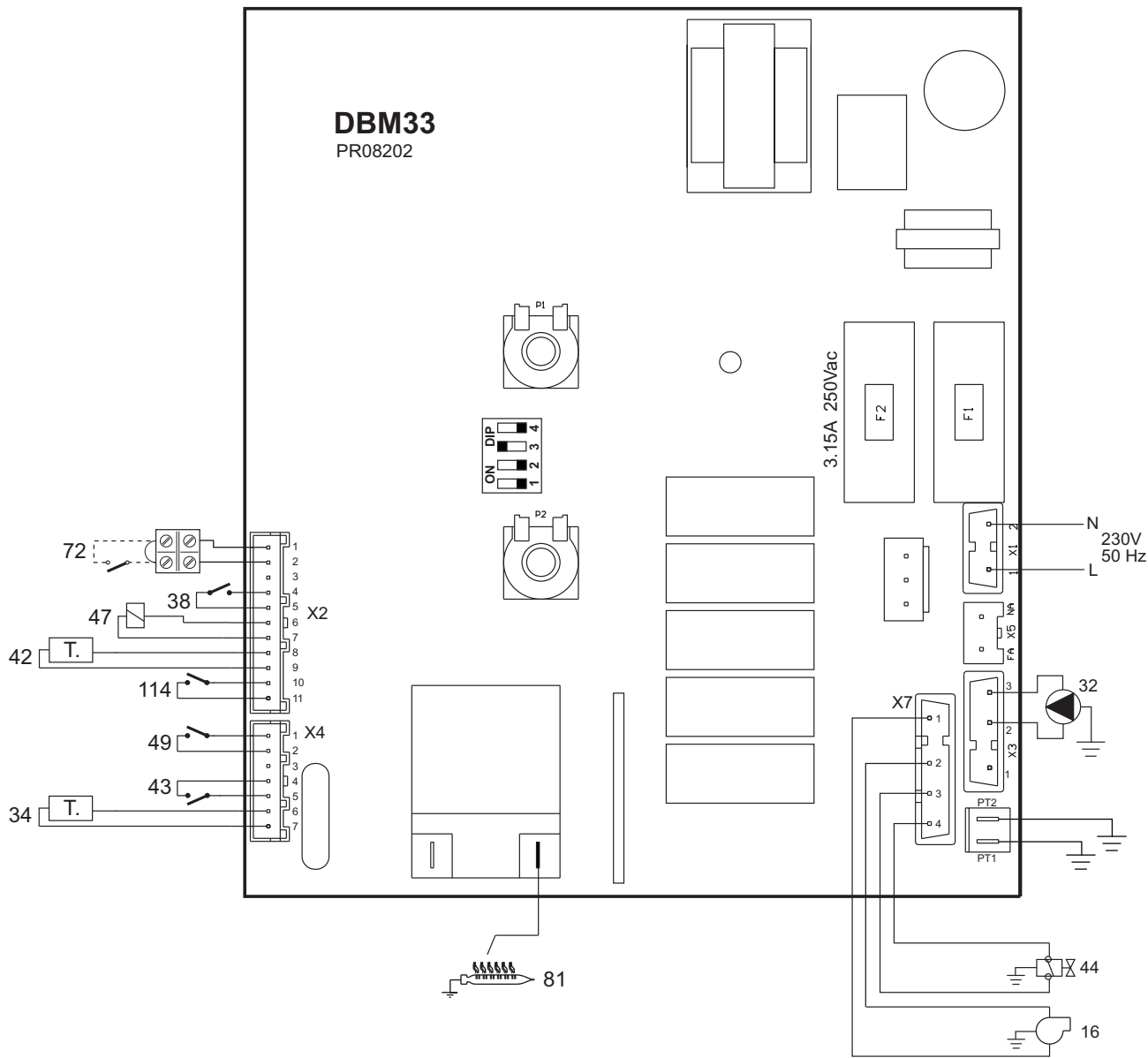
рис. 20 - Электрическая схема
