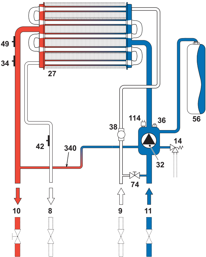
рис. 18 - Отопительный контур
