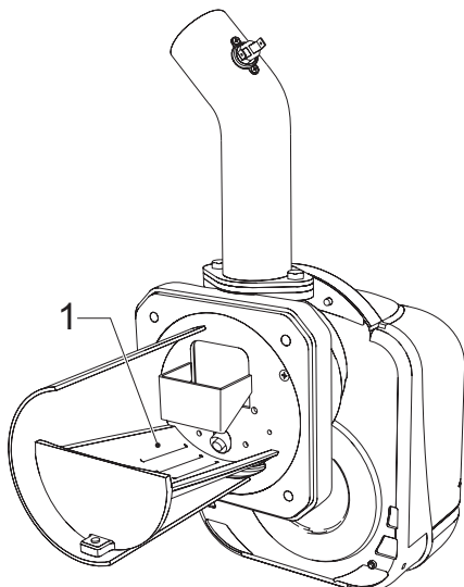
рис. 12 - Решетка горелки
